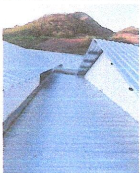
Foto 1: CUBIERTA DE LÁMINA Sustitución de techo de lámina en mal estado por lámina troquelada calibre 26 en el área de los baños, área de pila y comedor. Sustitución de
